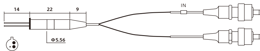
パッケージ概略図
