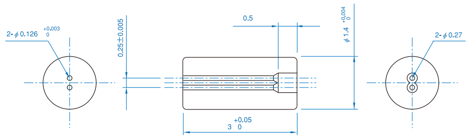
二芯キャピラリー φ1.4mm
