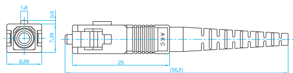
Fiber Cable Φ2.0mm
